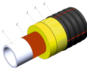
Рис. 1.2 - Конструкция ГПИ-трубы ИЗОКОМ РЕ-Ха до 95/0,6/1,0 МПа
