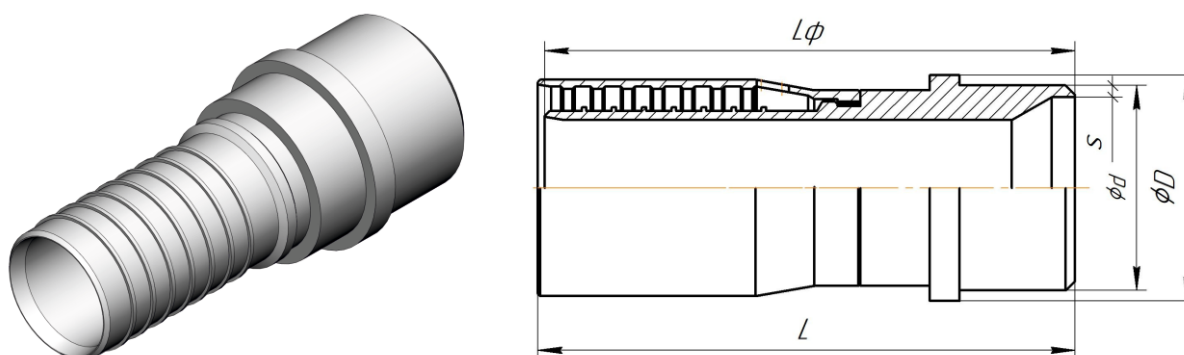
Фитинг обжимной под сварку
