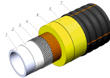
Рис. 1.3 - Конструкция ГПИ-трубы ИЗОКОМ А-РЕ-Ха 115/1,0 МПа ИЗОКОМ А-РЕ-Ха 115/1,6 МПа ИЗОКОМ А-РЕ-Ха 120/1,0 МПа
