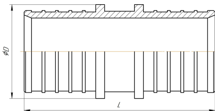
Пресс-муфта равнопроходная
