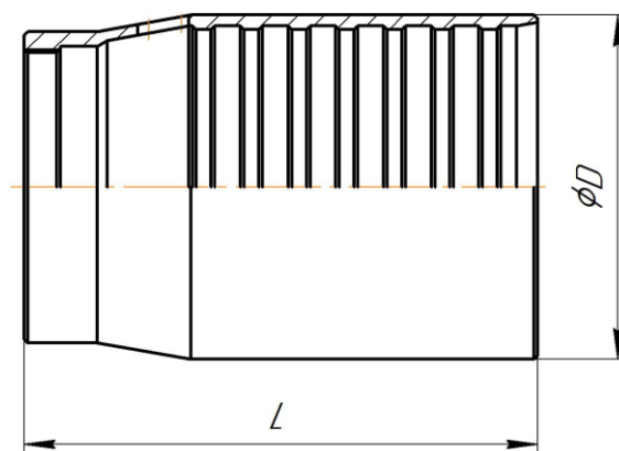
Гильза обжимная
