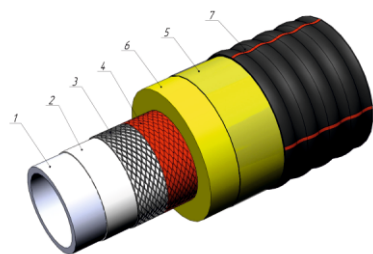
Рис. 1.1 - Конструкция ГПИ-трубы ИЗОКОМ А-РЕ-RT тип II 75/1,0 МПа ИЗОКОМ А-РЕ-Ха 95/1,0 МПа
