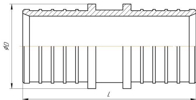
Пресс-муфта равнопроходная
